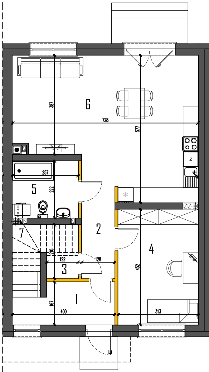
RZUT PARTERU
