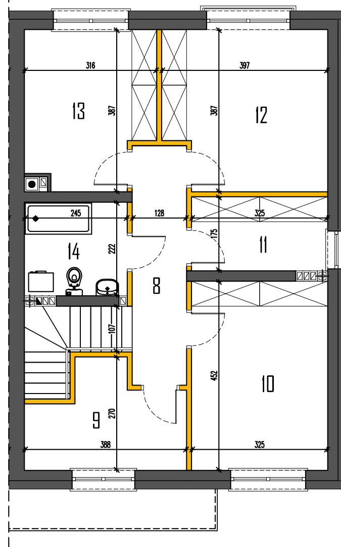
RZUT PIĘTRA
